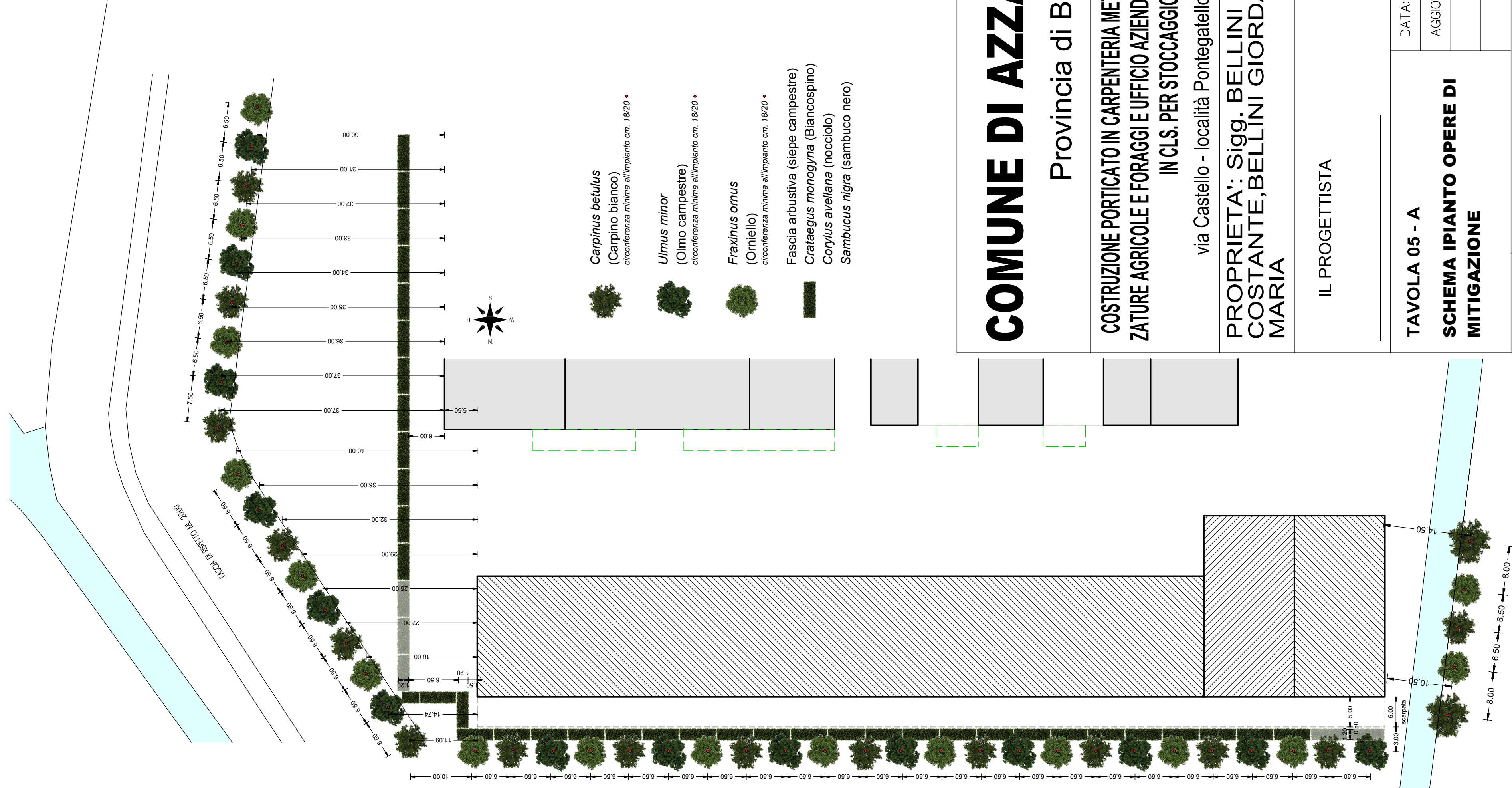
SCHEMA OPERE DI MITIGAZIONE - PLANIMETRIA 1:500
